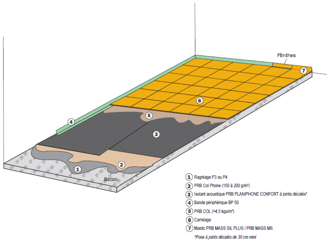
Figure 1b – Principe de pose du système PRB PLANIPHONE CONFORT en locaux P2 E1 / E2 avec PRB COL FLUID HPR
