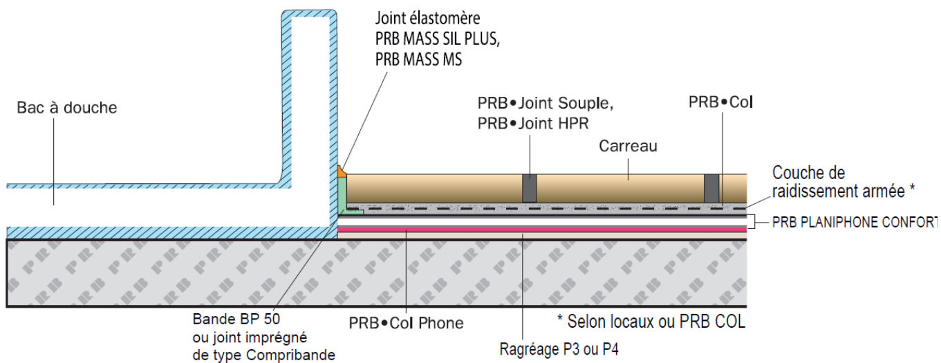
Figure 2 – Traitement d'un raccord avec bac à douche sur support maçonné en association avec PRB COL FLUID N
