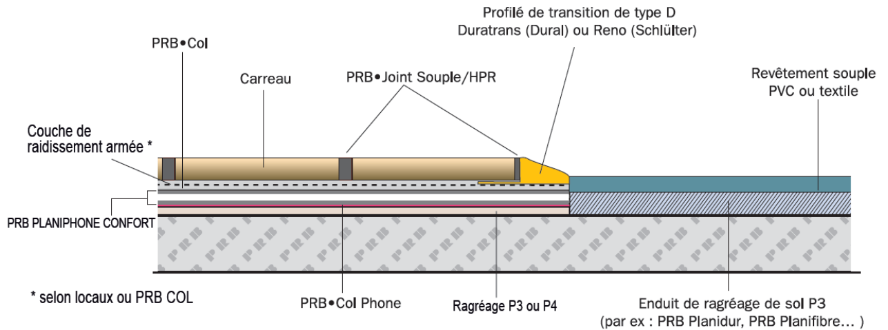
Figure 6 – Traitement d'un raccord entre le système PRB PLANIPHONE CONFORT et un revêtement de sol souple
