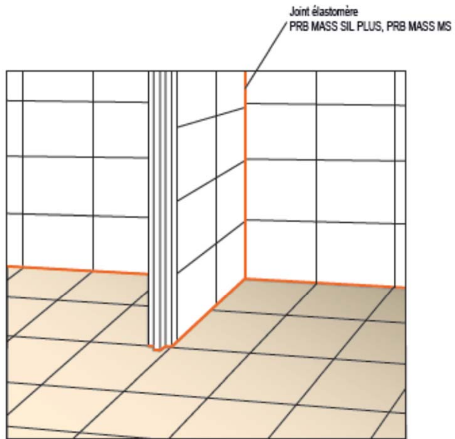
Figure 10 – Traitement des pieds d'huisseries et des angles sol-mur, mur-mur en locaux humides
