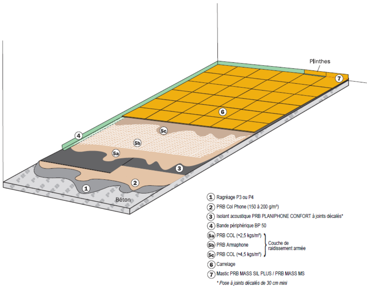
Figure 1a – Principe de pose du système PRB PLANIPHONE CONFORT avec ARMAPHONE
