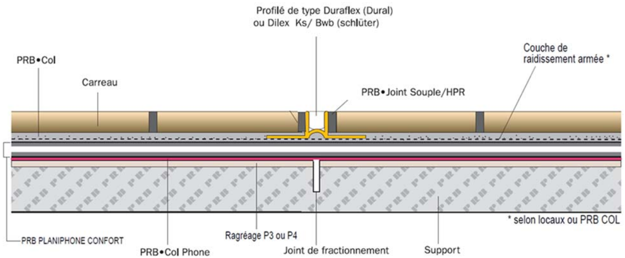
Figure 8 – Traitement des seuils de porte
