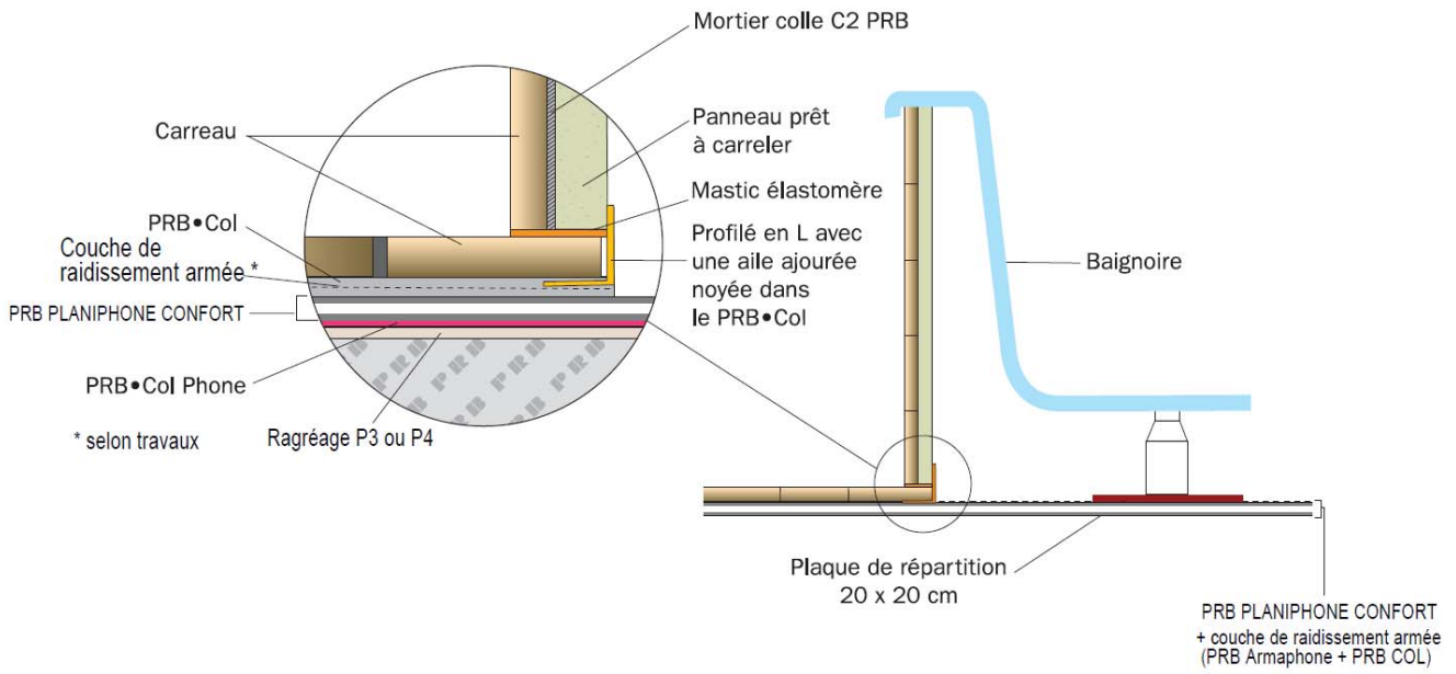
Figure 3 – Traitement d'un raccord avec une allège non maçonnée (sur support maçonné)
